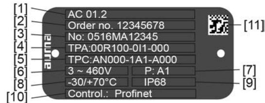
Figure 6 : Plaque signalétique de la commande de servomoteur (exemple)
