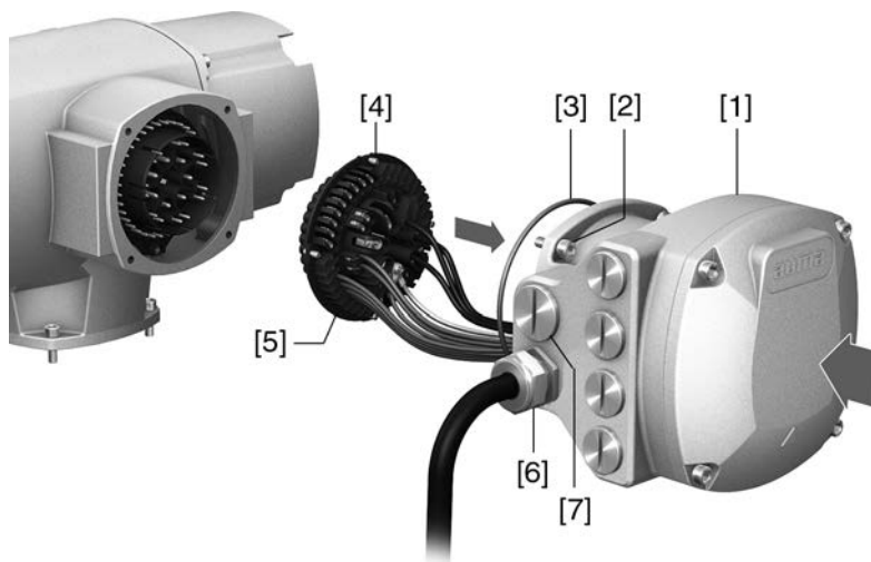
Figure 21 : Fermer la boîte de raccordement secteur
