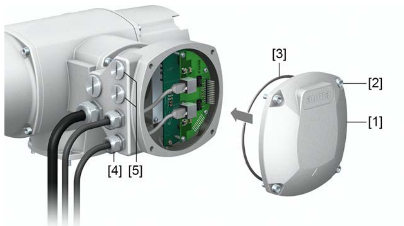
Figure 26 : Fermer la boîte de raccordement bus de terrain
