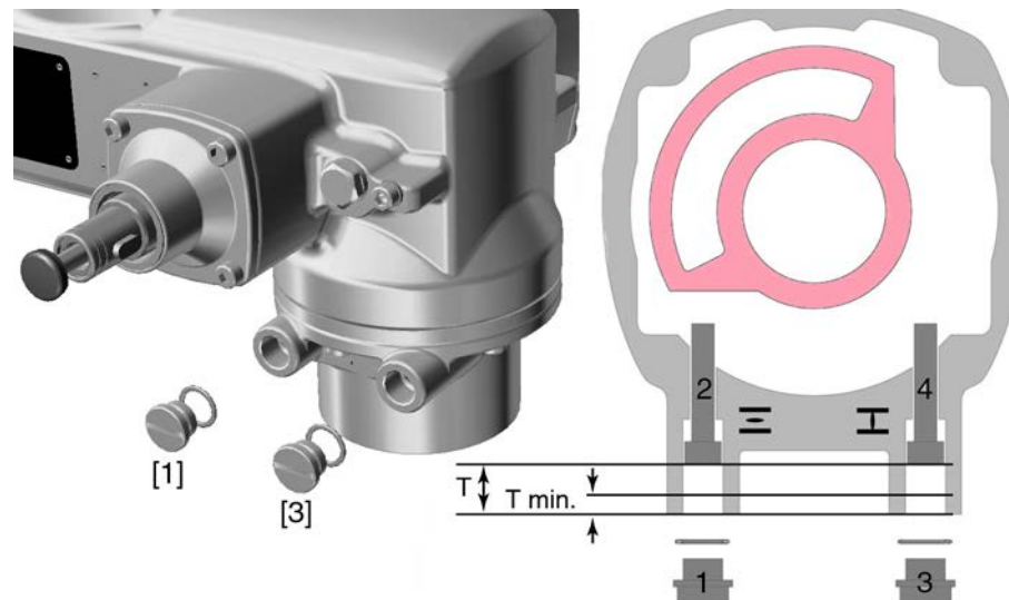
Figure 62 : Butée de position finale
