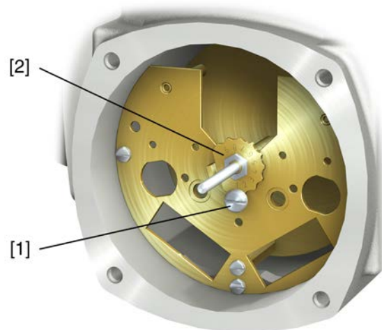
Figure 73 : Unité de commande avec réducteur
