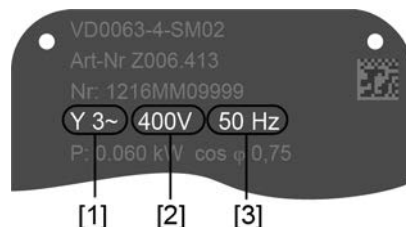
Figure 16 : Plaque signalétique moteur (exemple)
