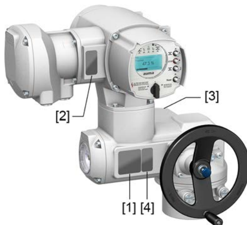
Figure 4 : Disposition des plaques signalétiques
