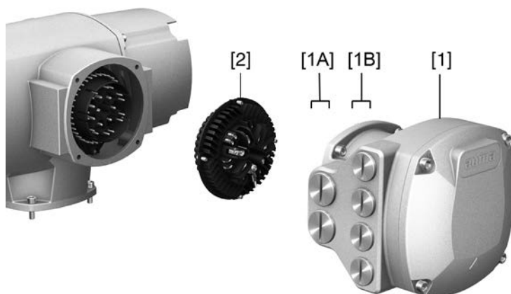
Figure 17 : Raccordement électrique SF
