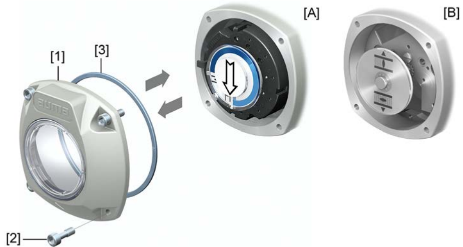
Figure 67 : Ouvrir/fermer le boîtier de commande
