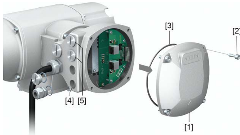
Figure 22 : Ouvrir le capot de la boîte de raccordement pour bus de terrain
