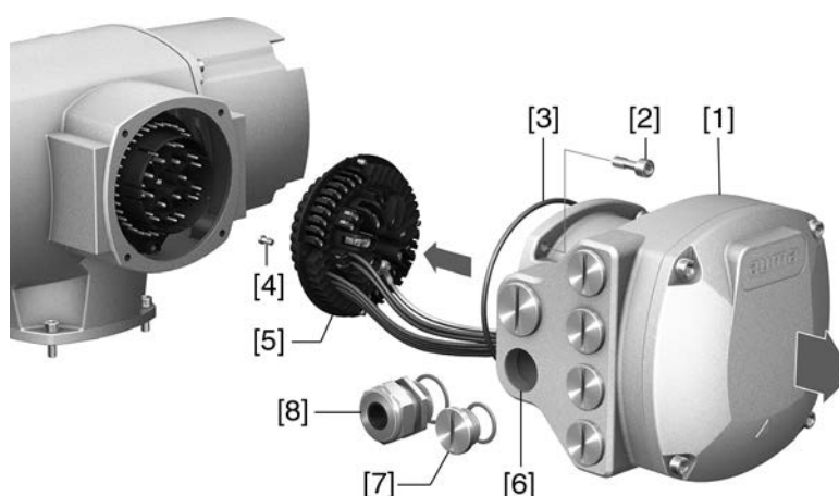
Figure 18 : Ouvrir la boîte de raccordement secteur
