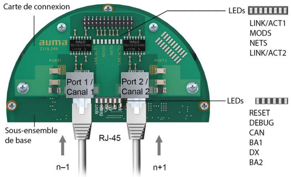
Figure 25 : Carte de connexion Profinet avec ces raccordements RJ-45
