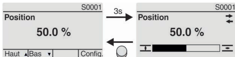
Figure 44 : Position de la vanne et affichage de la direction de manœuvre
