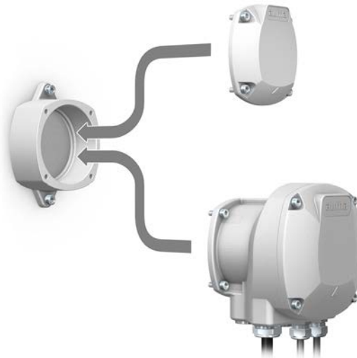
Figure 28 : Support temporaire, exemple avec multiconnecteur AUMA et capot
