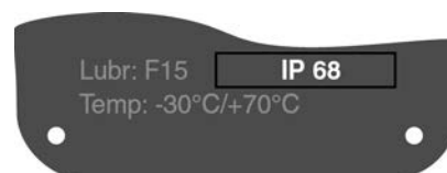
Figure 23 : Exemple : Plaque signalétique IP68
